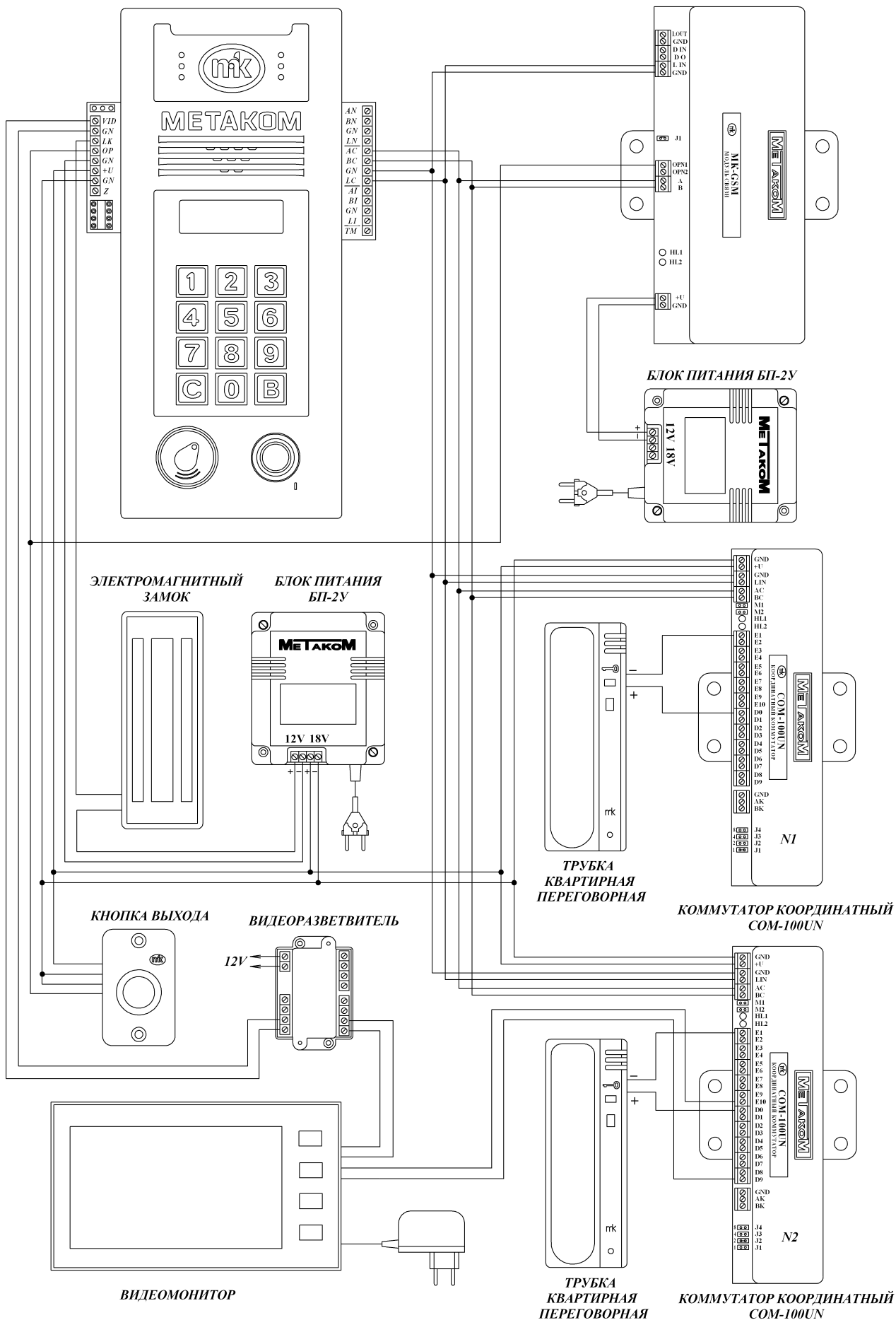
Рис. 2 Пример монтажа блока вызова МК2018-TMRFV
