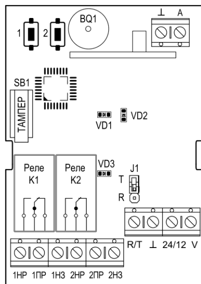
Рис.1 Плата приёмника «Лидер-4»
