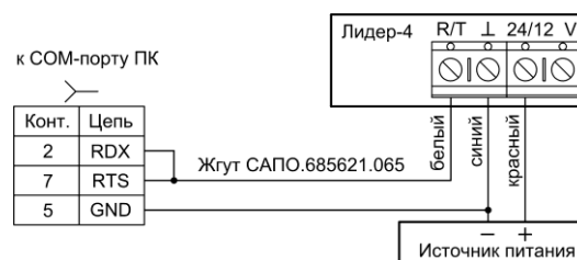
Рис.5 Схема подключения приёмника «Лидер-4» к COM-порту компьютера.
