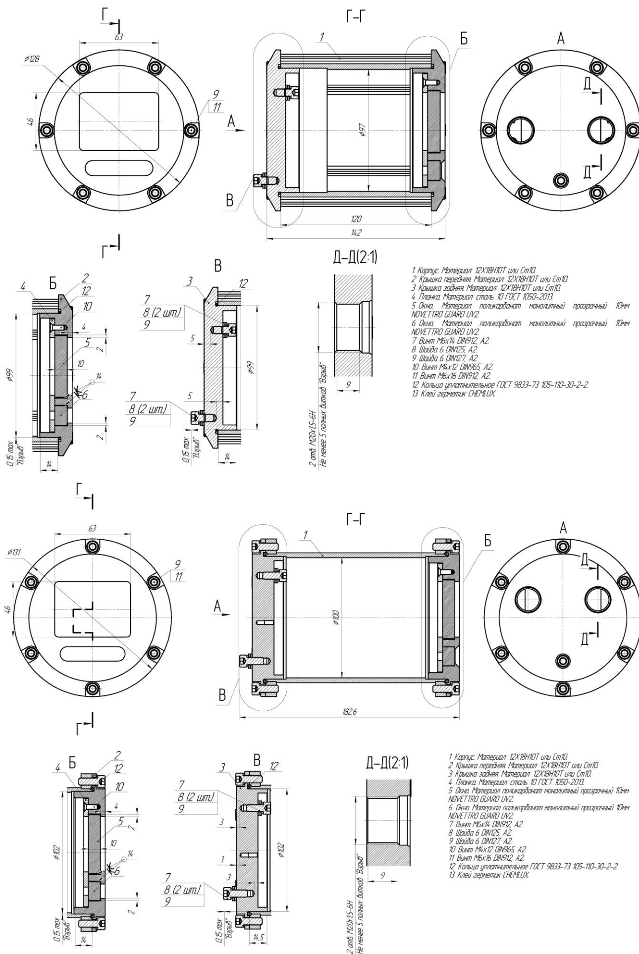
Рисунок А3 – Чертеж безопасности
