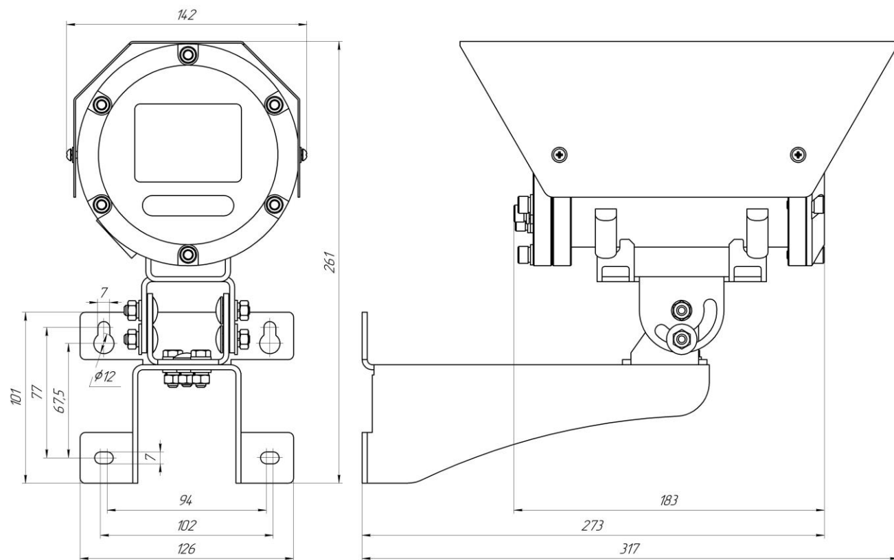
Рисунок А2 – Габаритные размеры видеокамеры ЗонЕкс-БК-Exd-H10, ЗонЕкс-БК-Exd-M10
