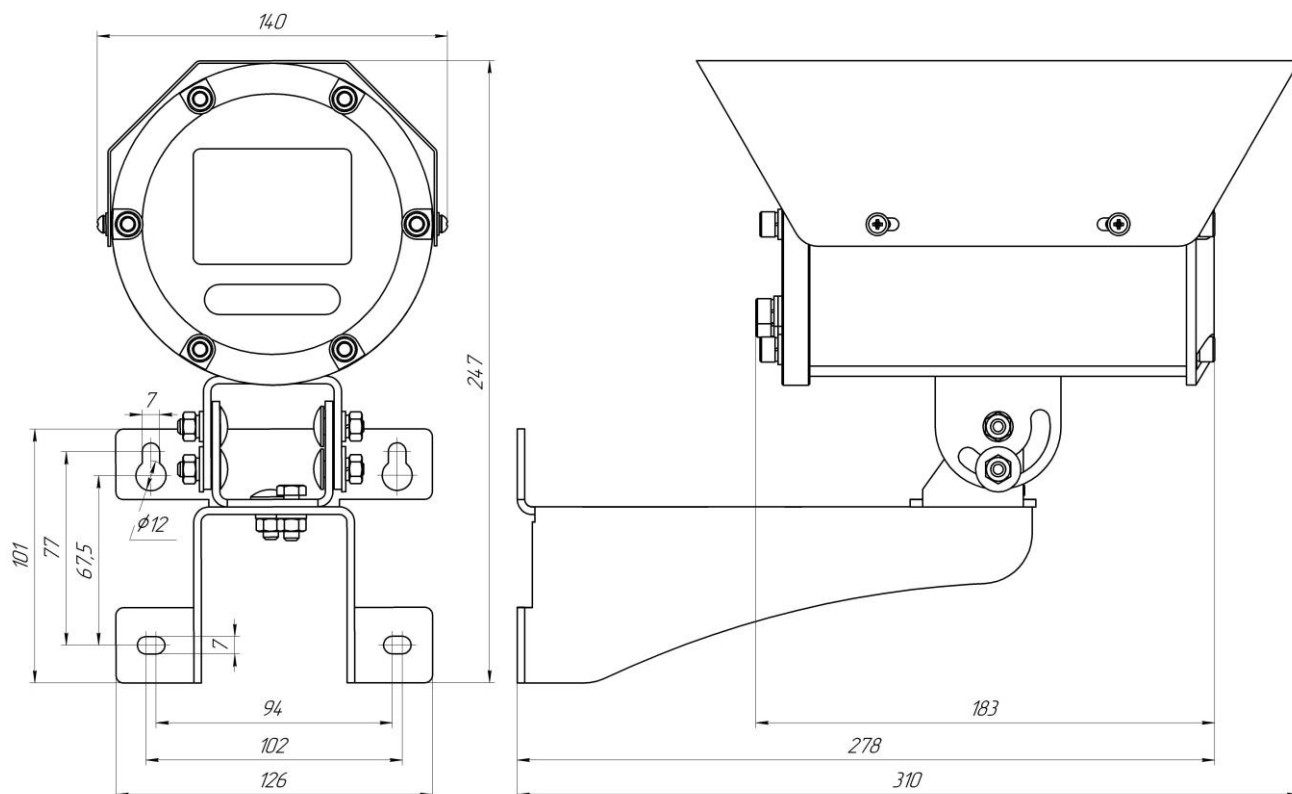
Рисунок А1 – Габаритные размеры видеокамеры ЗонЕкс-БК-Exd-A10
