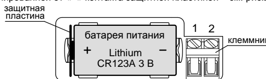
Рис.2 Батарейный отсек
