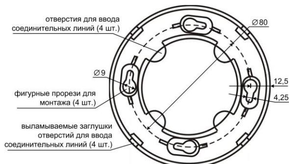
Рис.3 База извещателя. Присоединительные размеры
