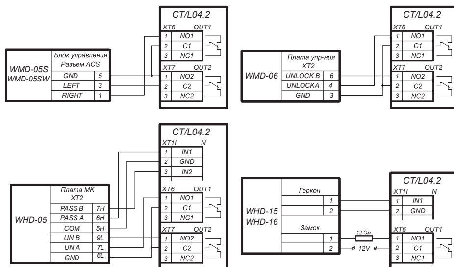
Схемы подключений калиток
