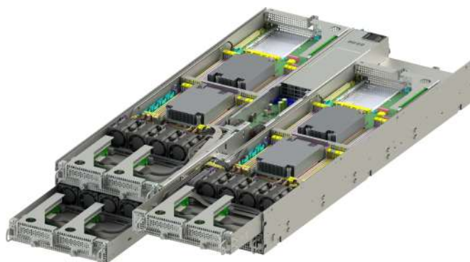
Сервер ПАЛАДИН-МШУ (тип 2) / Изометрия спереди без верхней крышки
